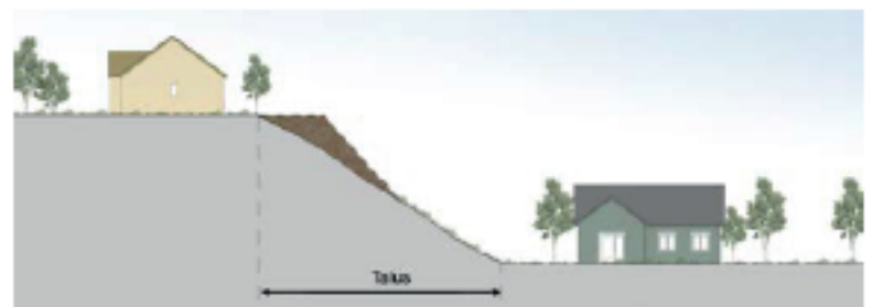
Figure 10 | Exemple de remblai visé par le cadre normatif
